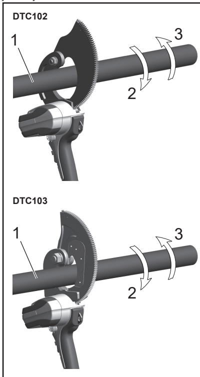
► 1. Kabel 2. Rotace řezání 3. Reverzní rotace
