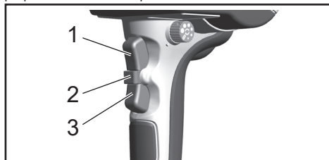
► 1. Çelësi i regjimit përpara 2. Bllokuesi i çelësit 3. Çelësi i regjimit të kthimit mbrapsht
