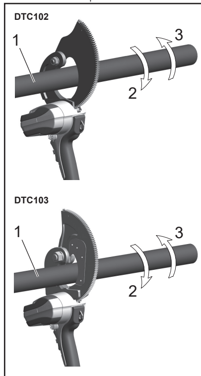
► 1. Cablu 2. Direcția de rotire pentru tăiere 3. Rotire înapoi
